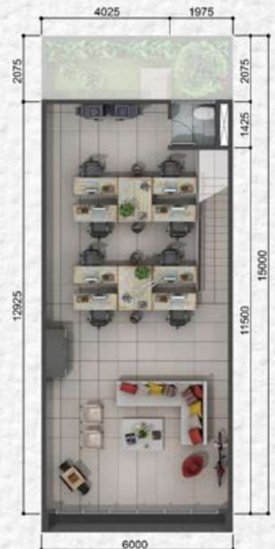
Lantai 3
